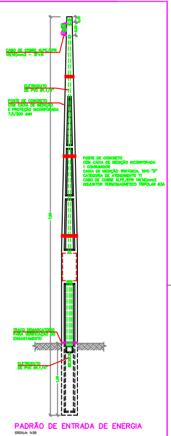
PADRÃO DE ENTRADA DE ENERGIA
