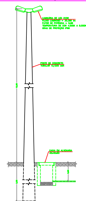
DETALHE DO POSTE DE ILUMINAÇÃO
